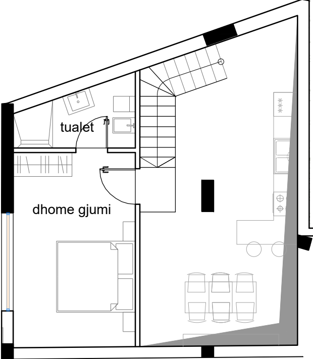
PLANIMETRIA E KATIT SIPER kuota +15.84
