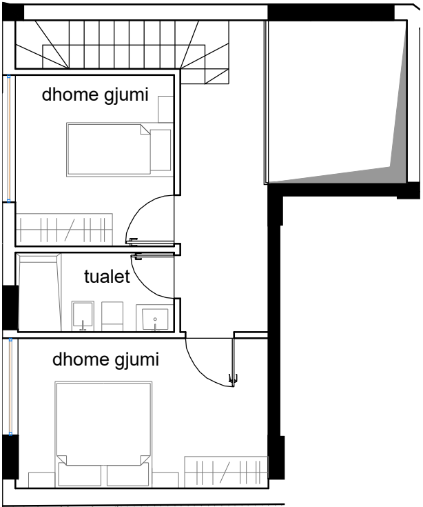
PLANIMETRIA E KATIT SIPER kuota +22.38
