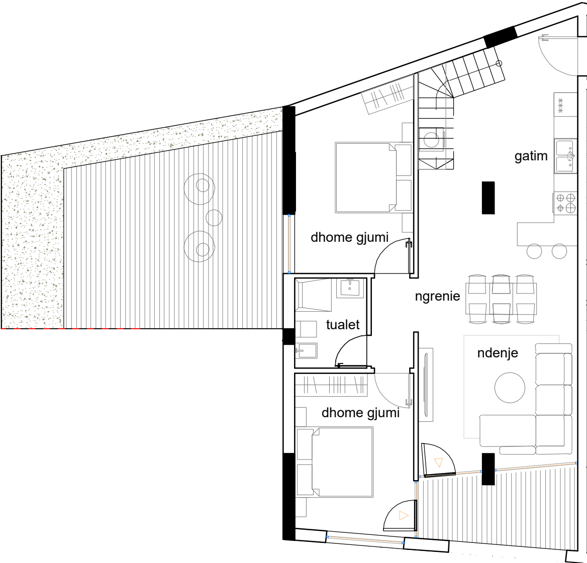
PLANIMETRIA E KATIT TE POSHTEM kuota +12.60
