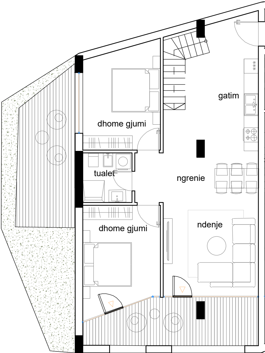
PLANIMETRIA E KATIT TE POSHTEM kuota +12.60
