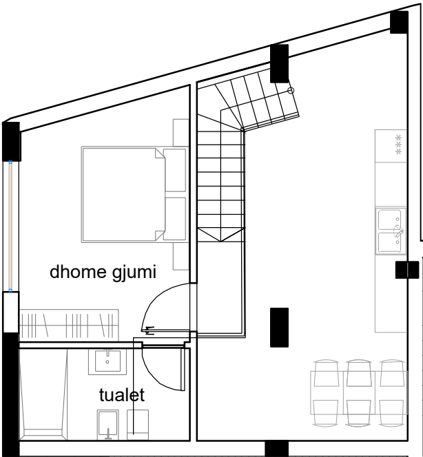
PLANIMETRIA E KATIT SIPER kuota +15.84
